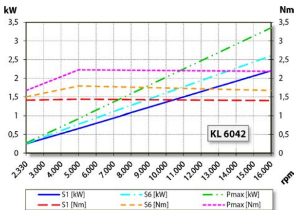
Vermogensdiagram
