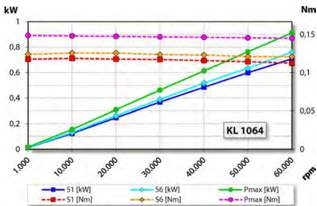
Diagram výkonu Chlazení nosiče vřeten
