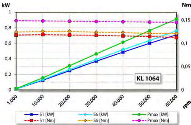
성능 다이어그램 스핀들 브래킷 냉각
