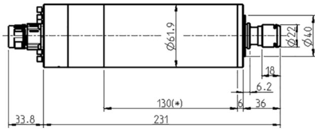
Abmessungen
