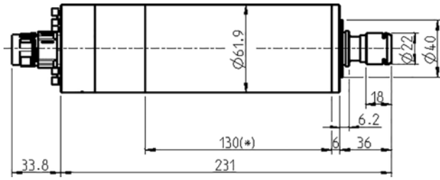
寸法図
