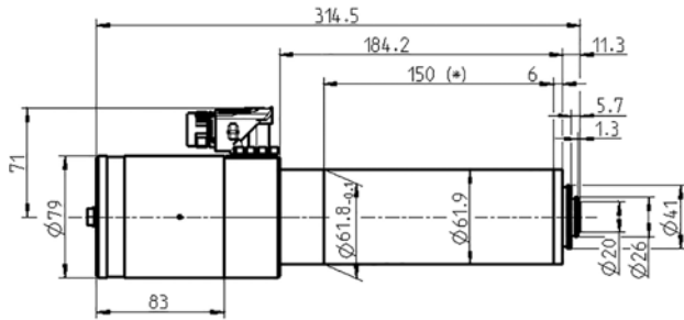
寸法図
