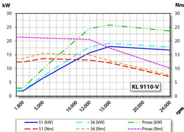
出力、トルク-回転数ダイアグラム
