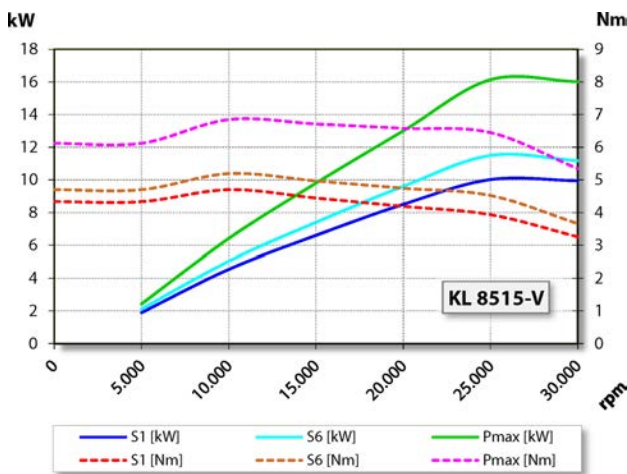
Diagram výkonu
